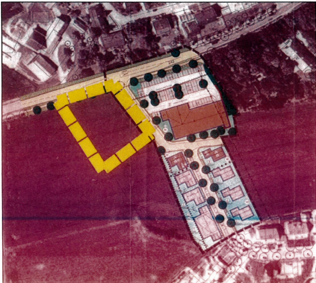
Bebauungs- und Grünordnungsplan „Lerchenau-Erweiterung I“ der Gemeinde Würth a. d. Isar mit Darstellung des Geltungsbereichs der Flächennutzungs- und Landschaftsplanänderung (gelb gestrichelt)
